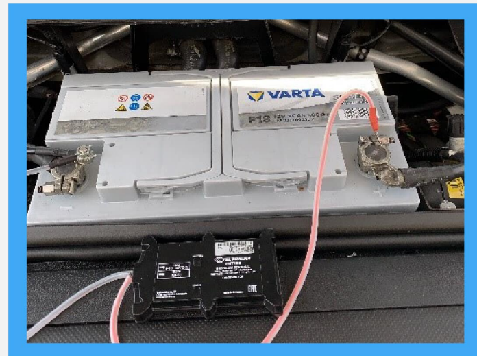
ÉTAPE 2: CONNECTEZ LES COSSES
